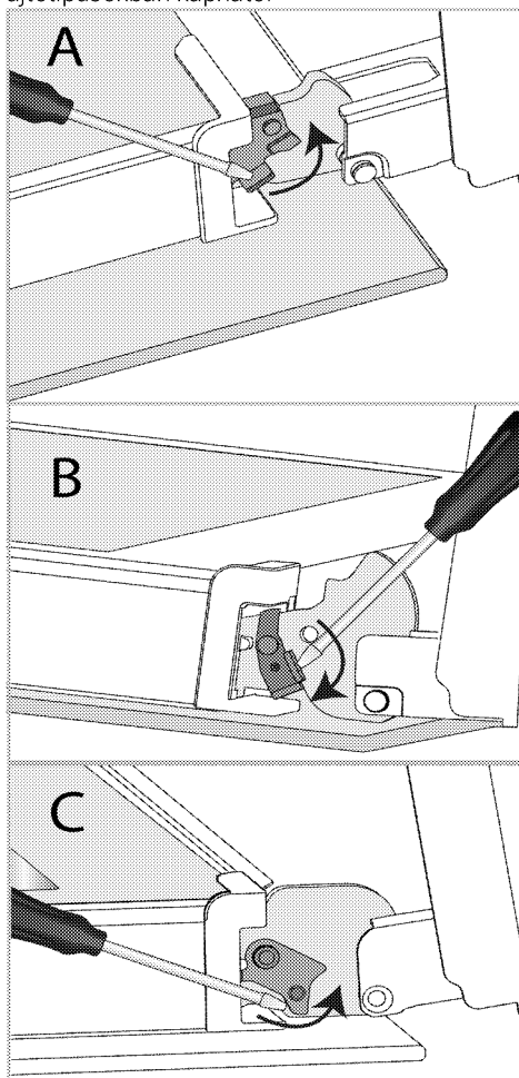
Zsanérzár - zárt helyzetben
