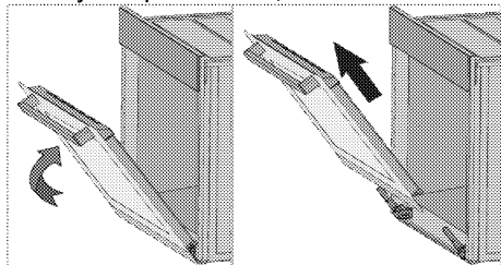
Заклучване на панти - отворено положение
