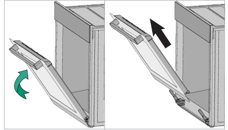
Çizim 6: Menteşe kilidi - açık pozisyon
