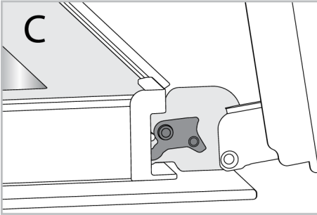
Çizim 6: Menteşe kilidi - açık pozisyon
