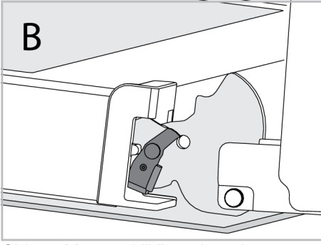
Çizim 4: Mentеше kilidi - açık pozisyon
