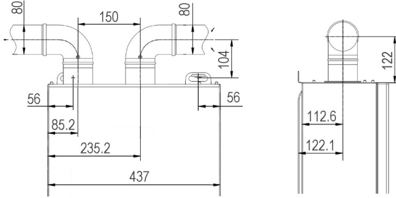
Şekil 28. 24/30/35 ikiz baca seti ölçüler
