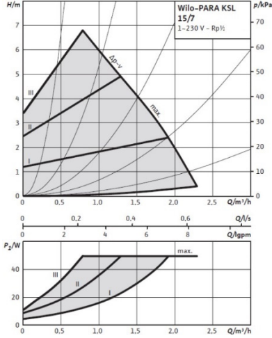
Değişken Basma Yüksekliği Eğrisi (Eğri 1)
