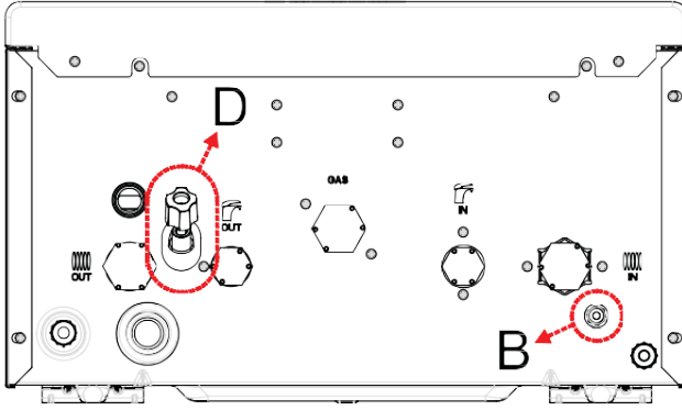
Şekil 3. Atria Pro kombi alttan görünüm
