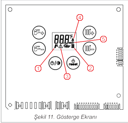
Şekil 11. Gösterge Ekranı
