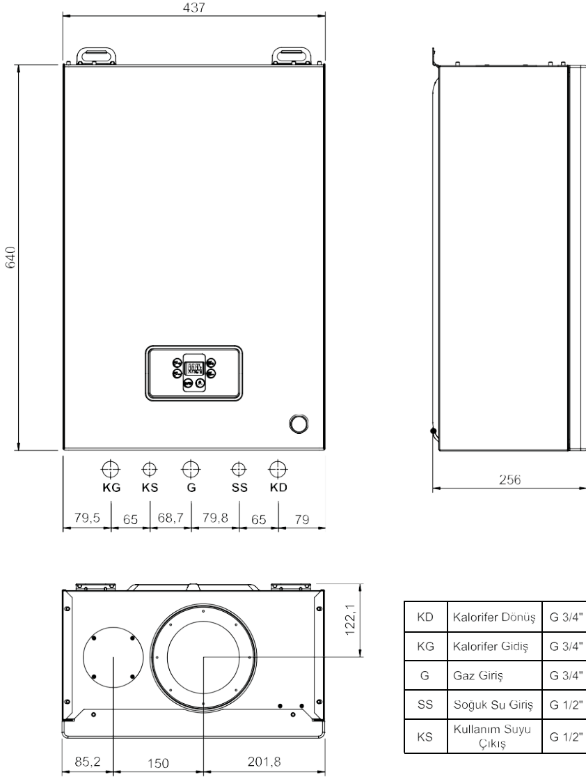
Şekil 6. Boyutlar
